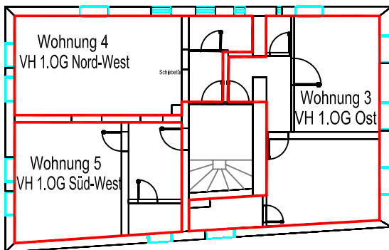
VH - 1.Obergeschoß
